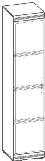
выс./шир./гл. 2126x444x440
