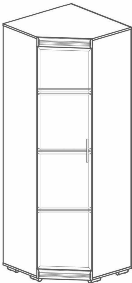
выс./шир./гл. 2126x740x417
