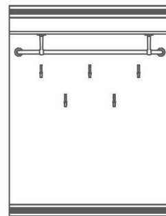
выс./шир./гл. 2186x1062x316
